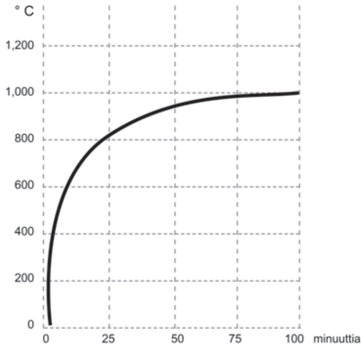
Kuvio 7. Tulipalon kehittymisen standardi-palokäyrä.
