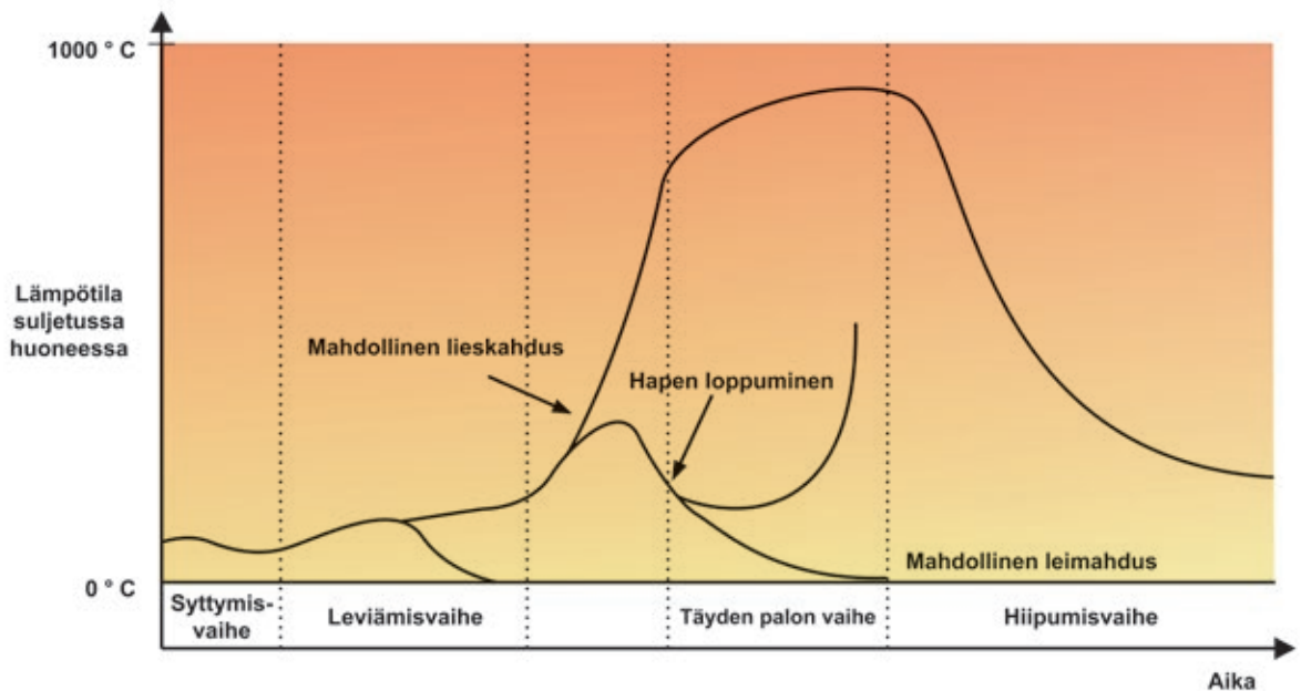
Kuvio 38. Palon eri vaihteita kuvaava palokäyrä.
