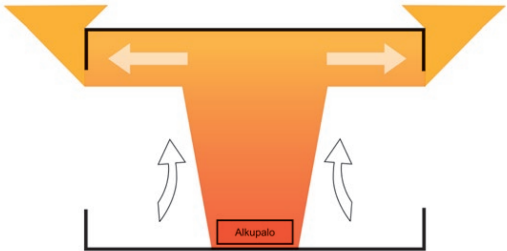
Kuvio 22. Polttoainerajoitteinen palo.
